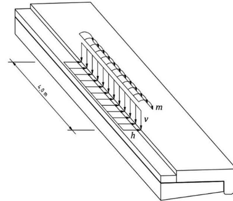
Bild 1 - Einwirkungen gemäß Tabelle 2 an der Schrammbordkante
